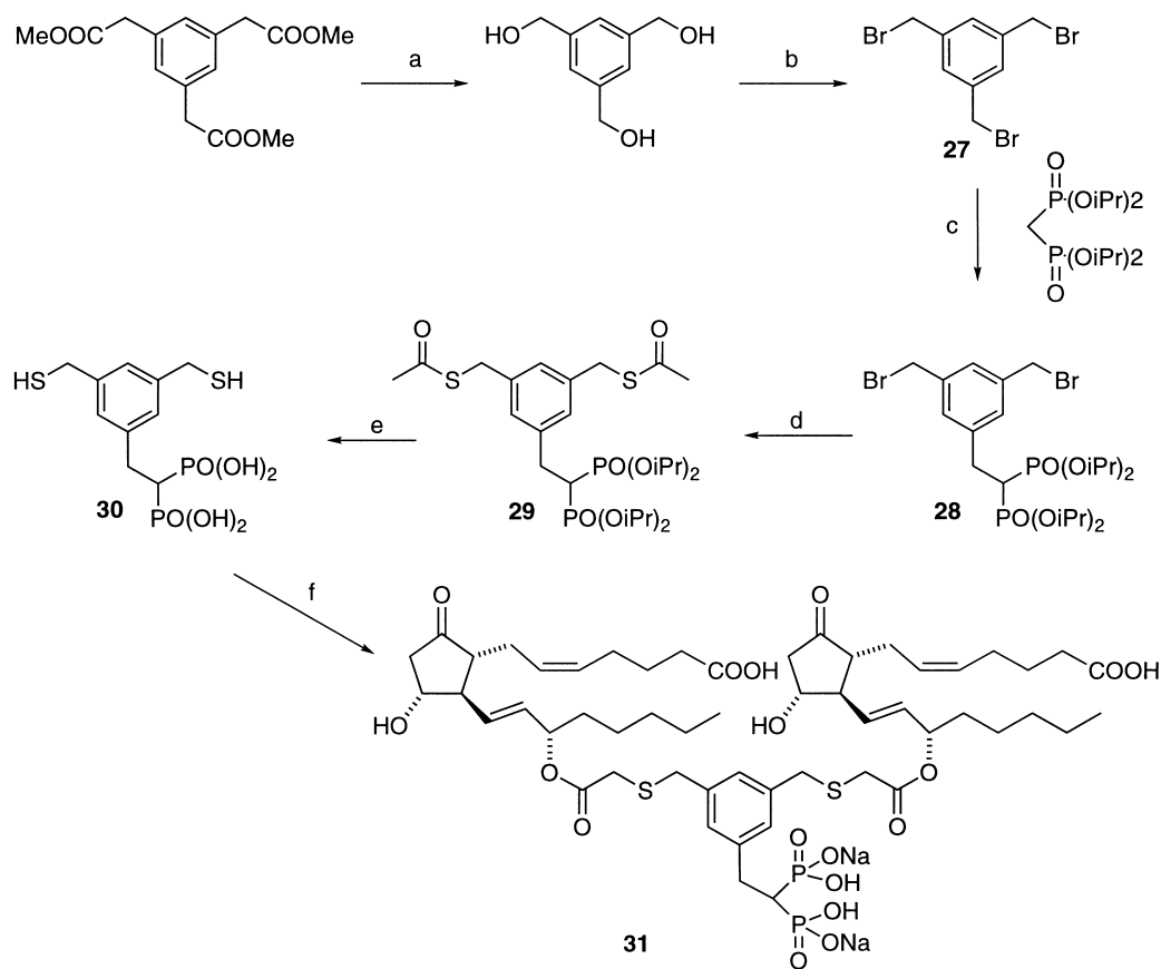
Scheme 7. Reagents: (a) \text{BH}_3\text{-SMe}_2 ; (b) \text{PBr}_3 ; (c) \text{NaH} , DMF; (d) \text{HSAc} , DMF; (e) \text{HCl} , reflux; (f) 1) 22 , \text{Et}_3\text{N} , dioxane, water. 2) \text{DOWEX}(\text{Na}^+) .
